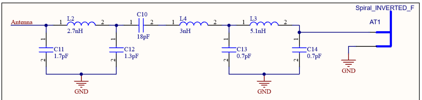
Figure 9.3. Antenna Path of BLE Module B1BMBG22M1
