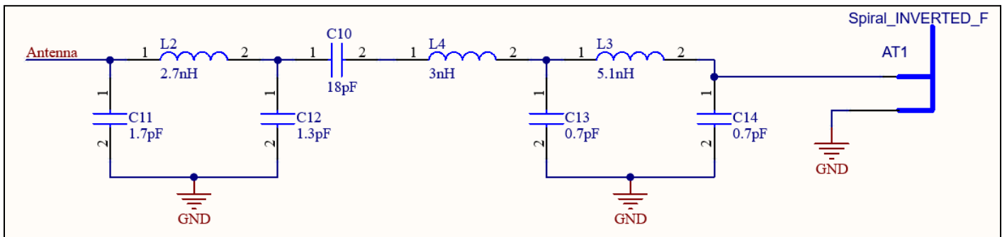
Figure 9.3. Antenna Path of BLE Module B1BMBG22M3
